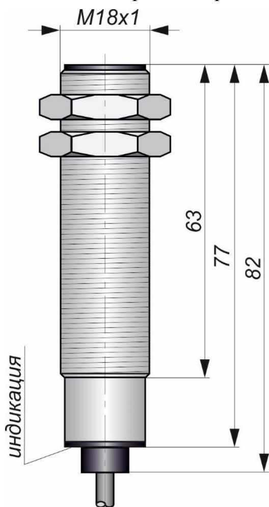
Габаритный чертеж
